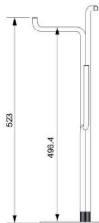
Papeleira Dupla de Chão
