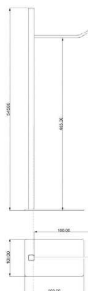
Papeleira de Chão Quadrado
