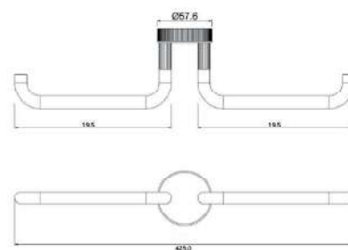
Porta Toalha Duplo
